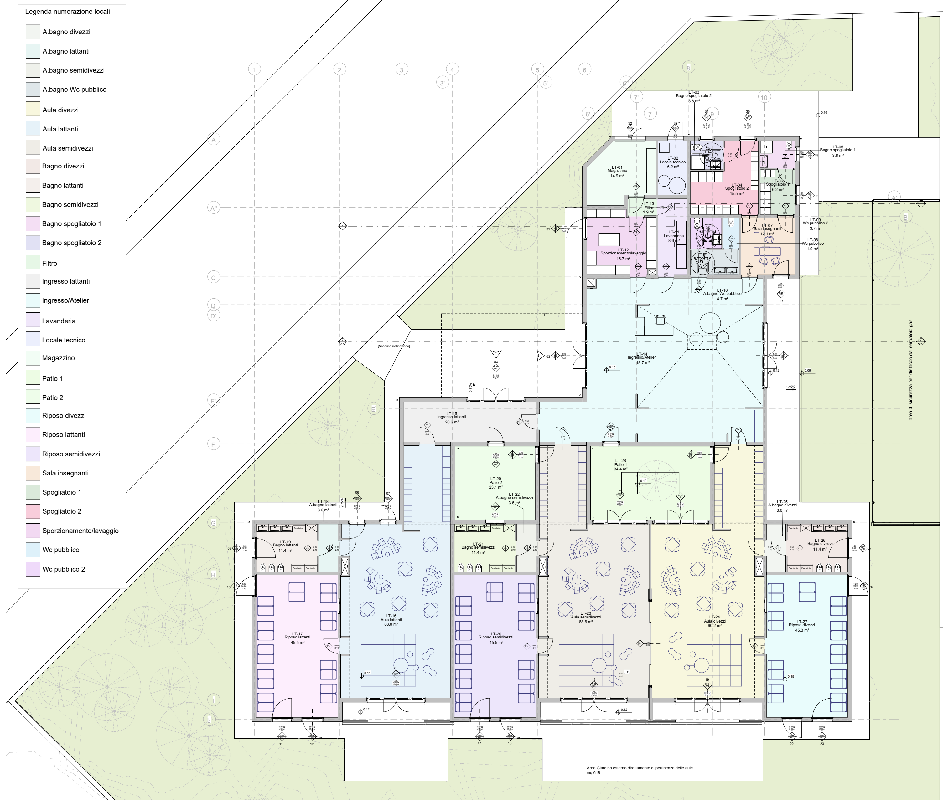
PIANTA ARREDATA PIANO TERRA SCALA 1:50
