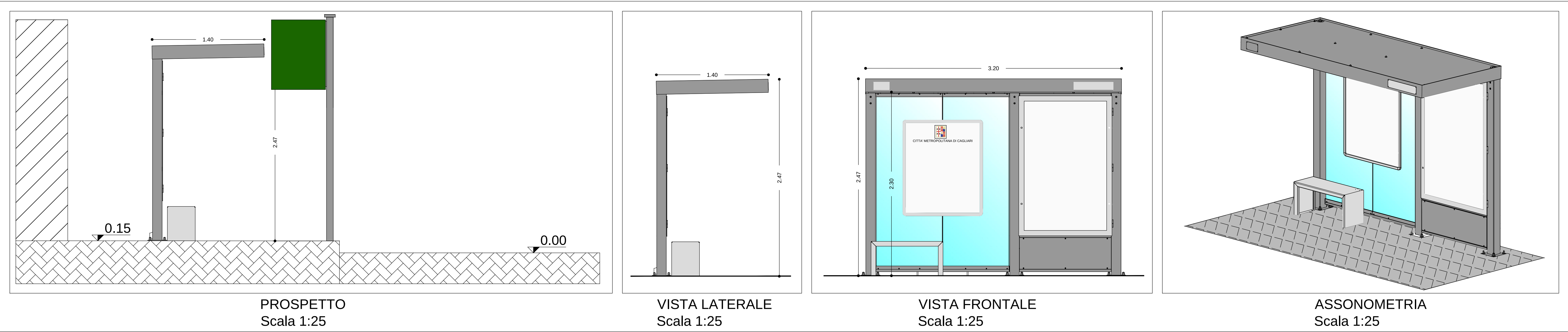
PENSILINA A SBALZO
