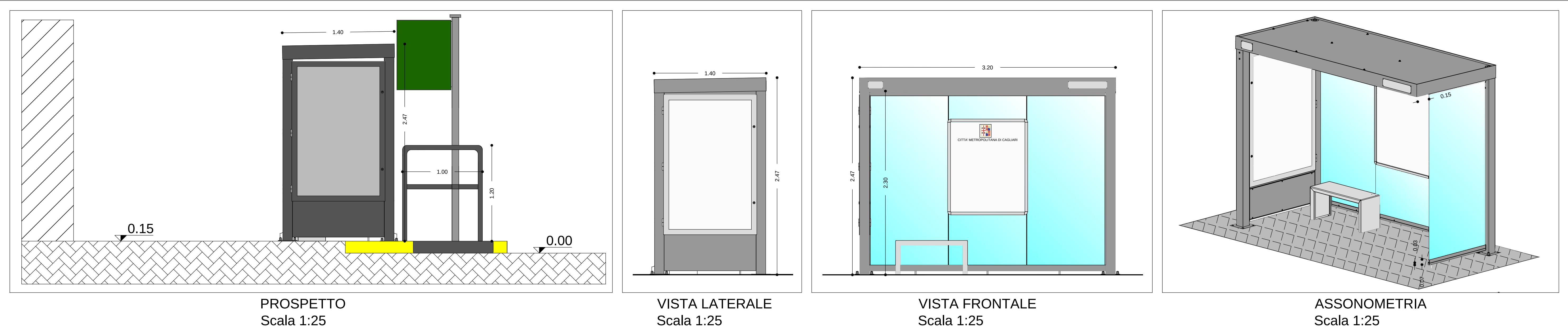
PENSILINA CON 3 MONTANTI
