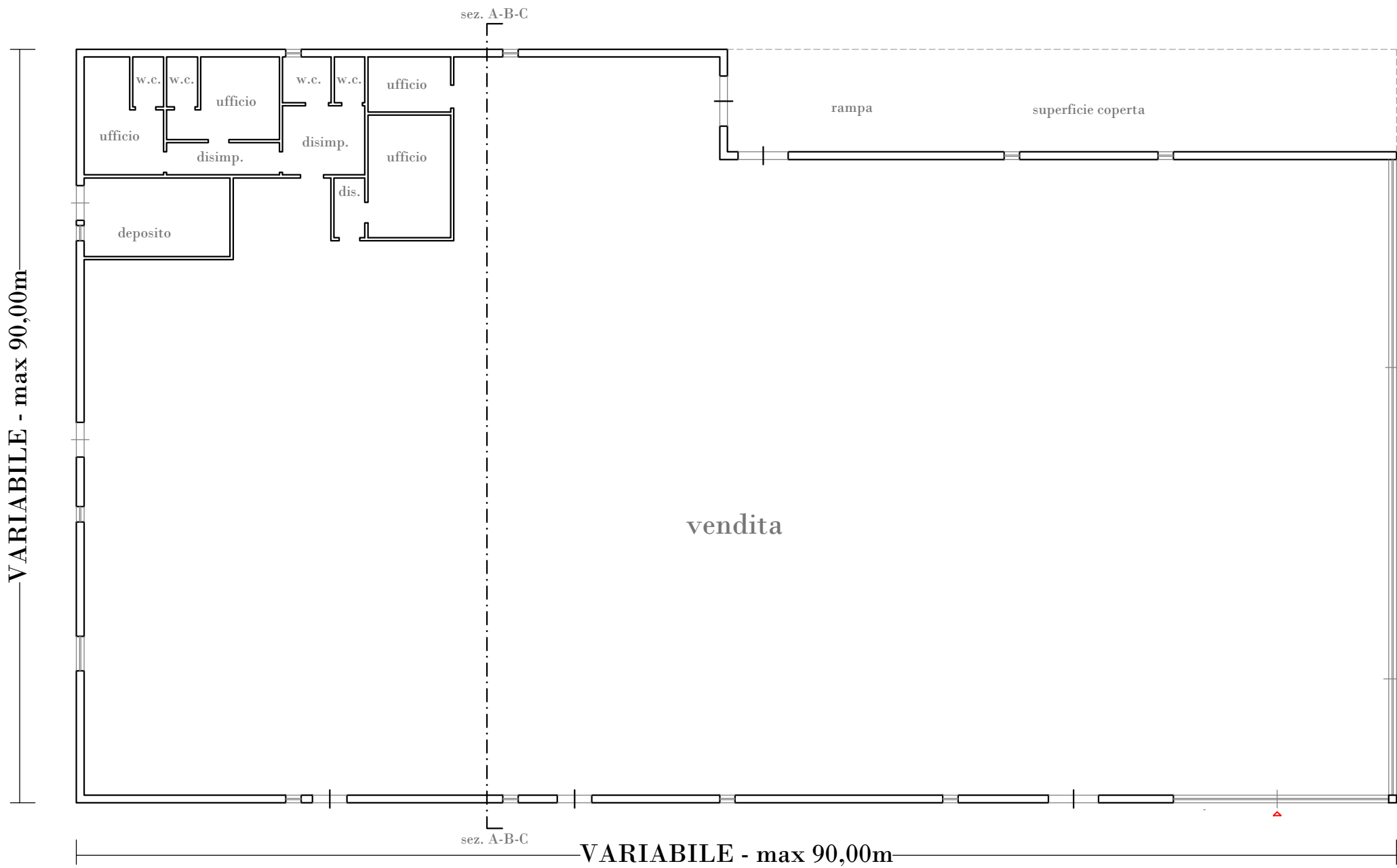
TIPOLOGIA 2 - MSV _ insediamento commerciale alimentare / non alimentare / misto - pianta piano terra - 1:200
