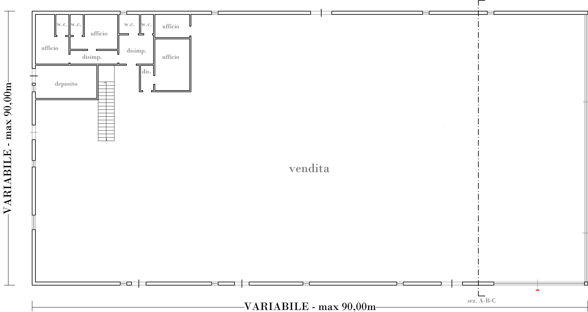
TIPOLOGIA 3 - UFFICI COMMERCIALI E LOCALI ESPOSITIVI - PIANO TERRA / PIANO PRIMO - 1:200
